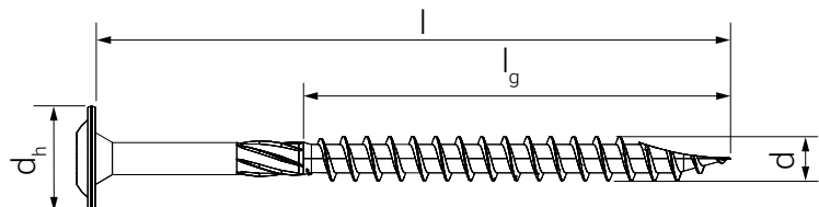
Abb. 2 STS-Schraube (Tellerkopf)
