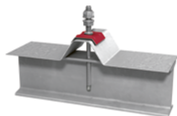
JT3-SB-3-8,0xL mit Dichtscheibe E16 + ORKAN-Kalotte für Trapezprofile
