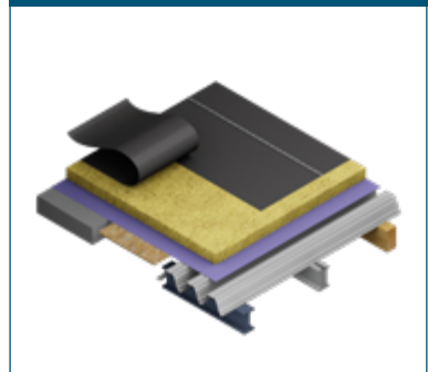
Flachdach mit Dichtungsbahn | siehe Seite 208
