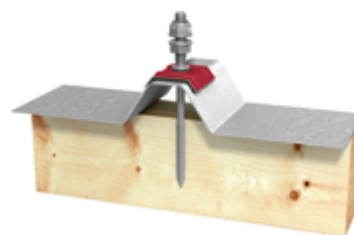
JA3-SB-8,0xL | JA3-SB-10,0xL mit Dichtscheibe E16 + ORKAN-Kalotte für Trapezprofile
