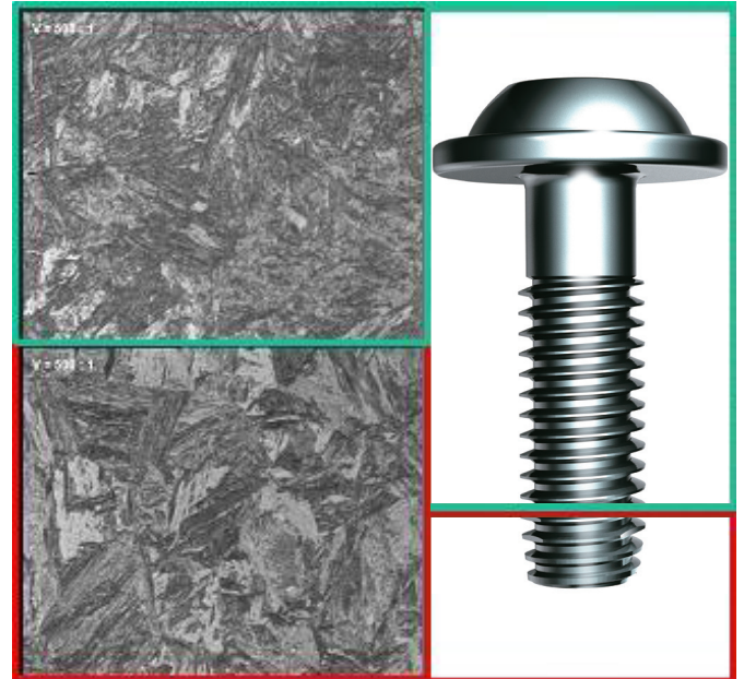
Gefügebau bei EJOT® HardTip Schrauben
